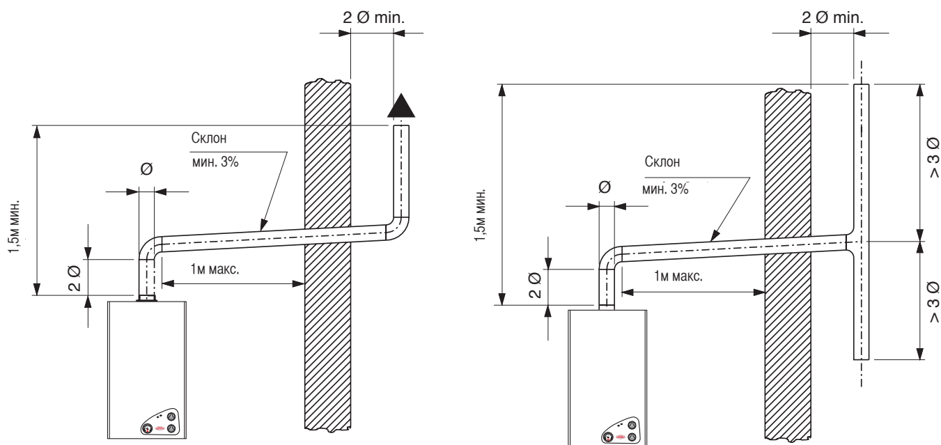
Рис. 9 – Подсоединение к дымоходу модели СТН
