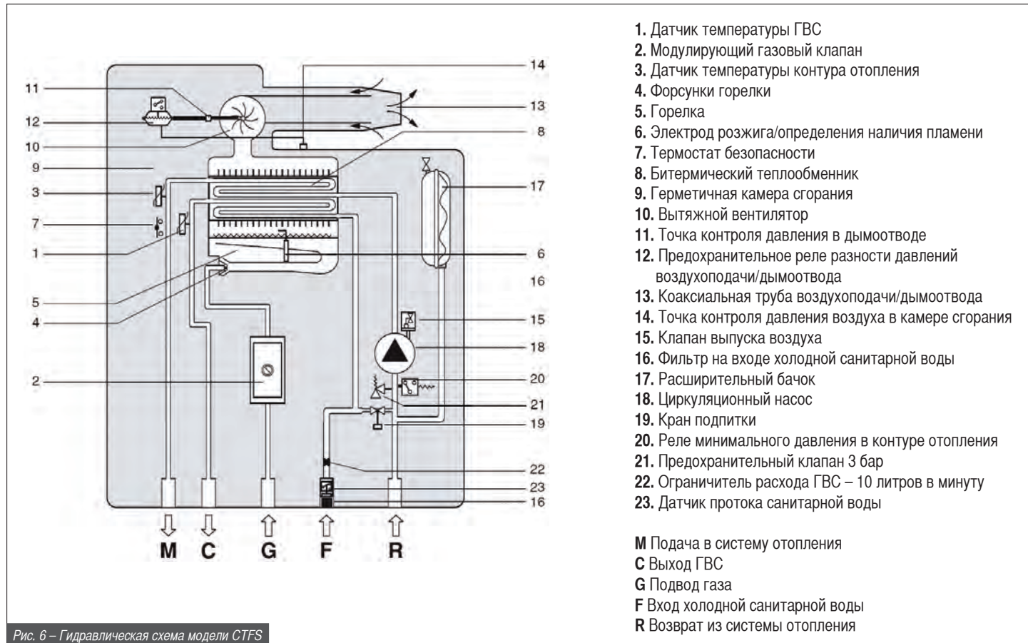
Рис. 6 – Гидравлическая схема модели СТФС
