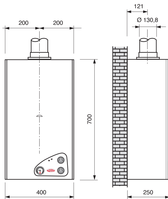
Рис.10 – Габаритные и разметочные размеры для подключения к дымоходу модели СТН
